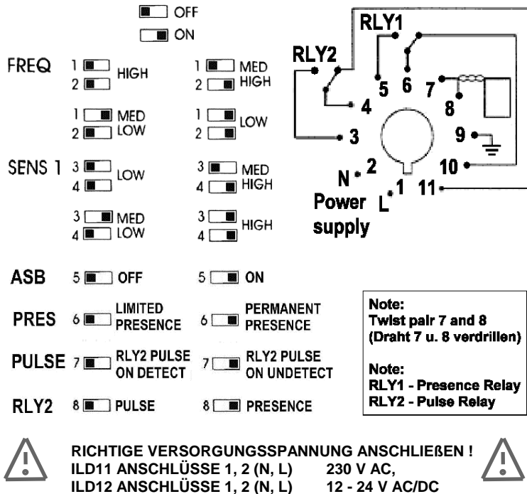
Bild 2 (Anschlussschema, s. auch seitlich am Gehäuse)
